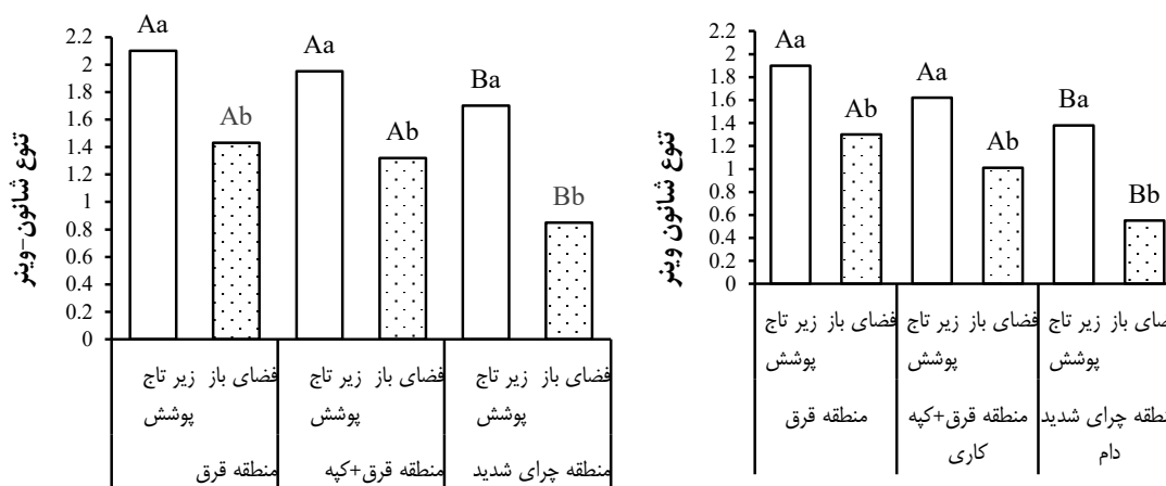
شکل ۳: مقایسه میانگین مقادیر شاخص تنوع شانون-وینر در زیر آشکوب گونه‌های پرستار و فضای مجاور (بین لکه‌ای) شکل سمت راست گونه Acantholimon raddeanum و شکل سمت چپ گونه Astragalus gossypinus Fisch. (حروف بزرگ، نشان‌دهنده معنی‌داری بین مکان‌ها و حروف کوچک، نشان‌دهنده معنی‌داری بین فضای باز و زیر آشکوب گونه در هر مکان)
